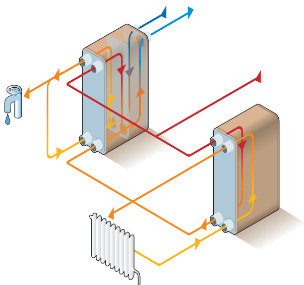
Двухступенчатое подключение
