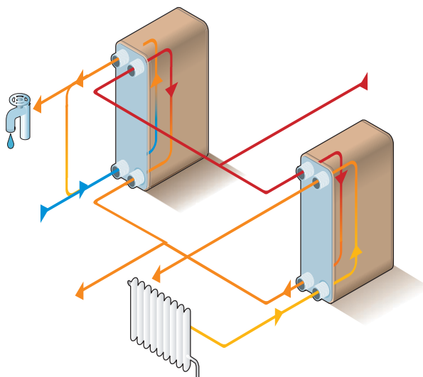
Параллельное подключение
